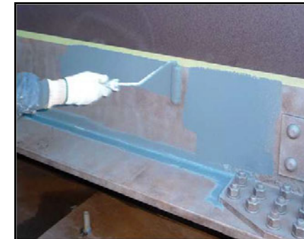
特殊有機ジンクリッチペイント塗布
