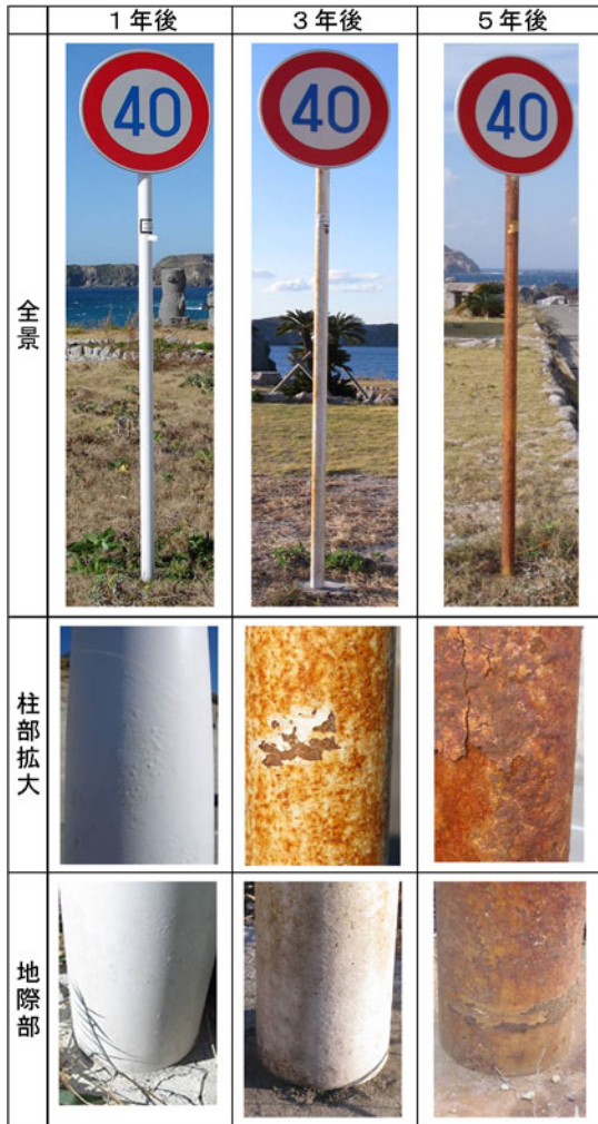
東京都新島村（平成17年11月試験建柱）
